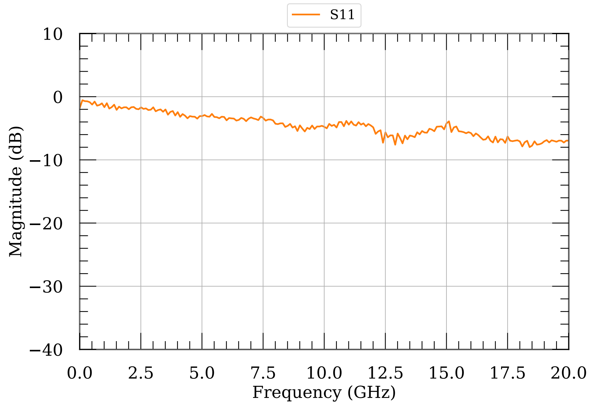
LNA S-params module080
